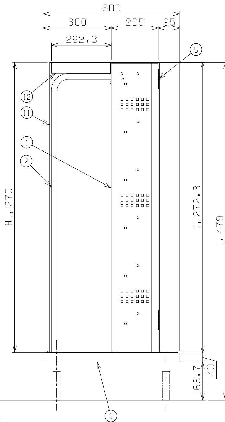
ツールリングホルダー詳細
