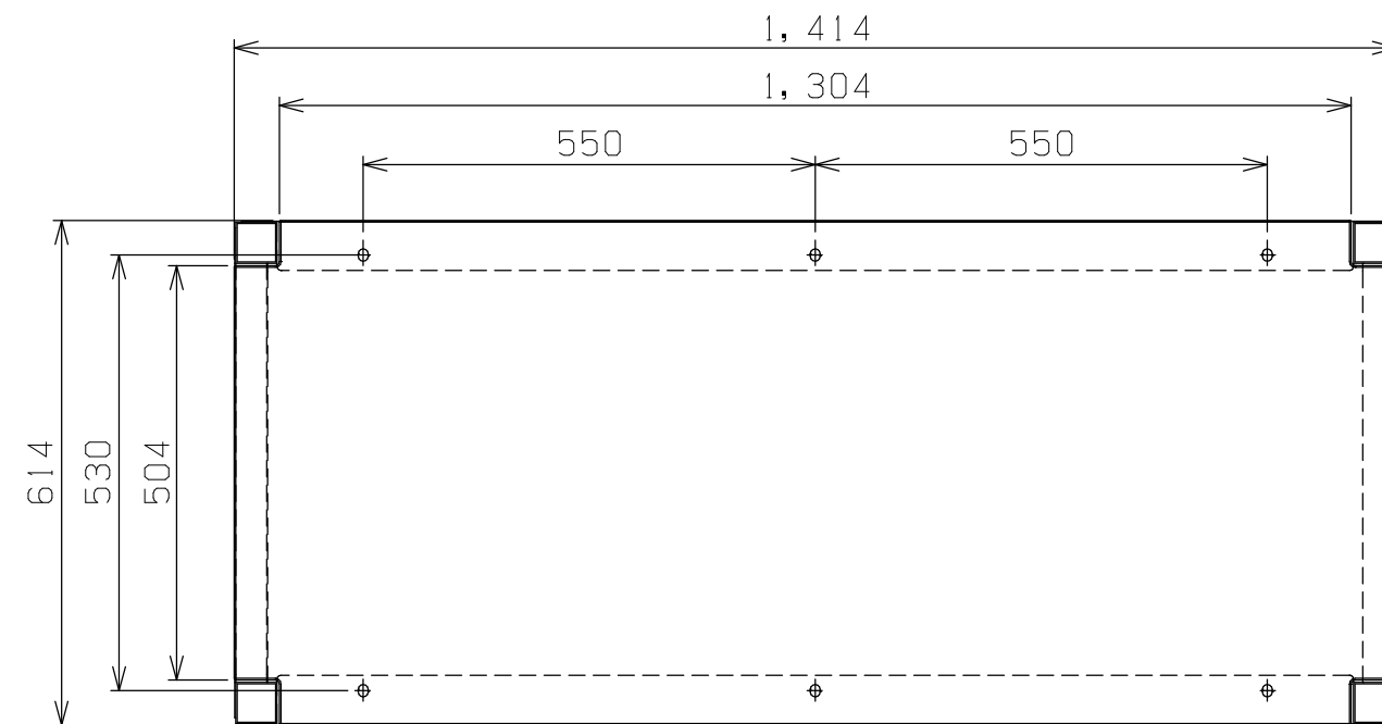
矢視A-A (S=1:10)
