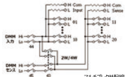
マルチプレクサ配線図
