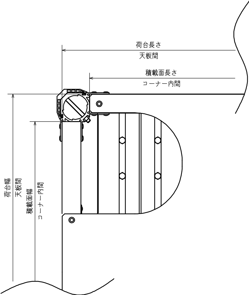
寸法詳細図 (S = 1 : 5)
