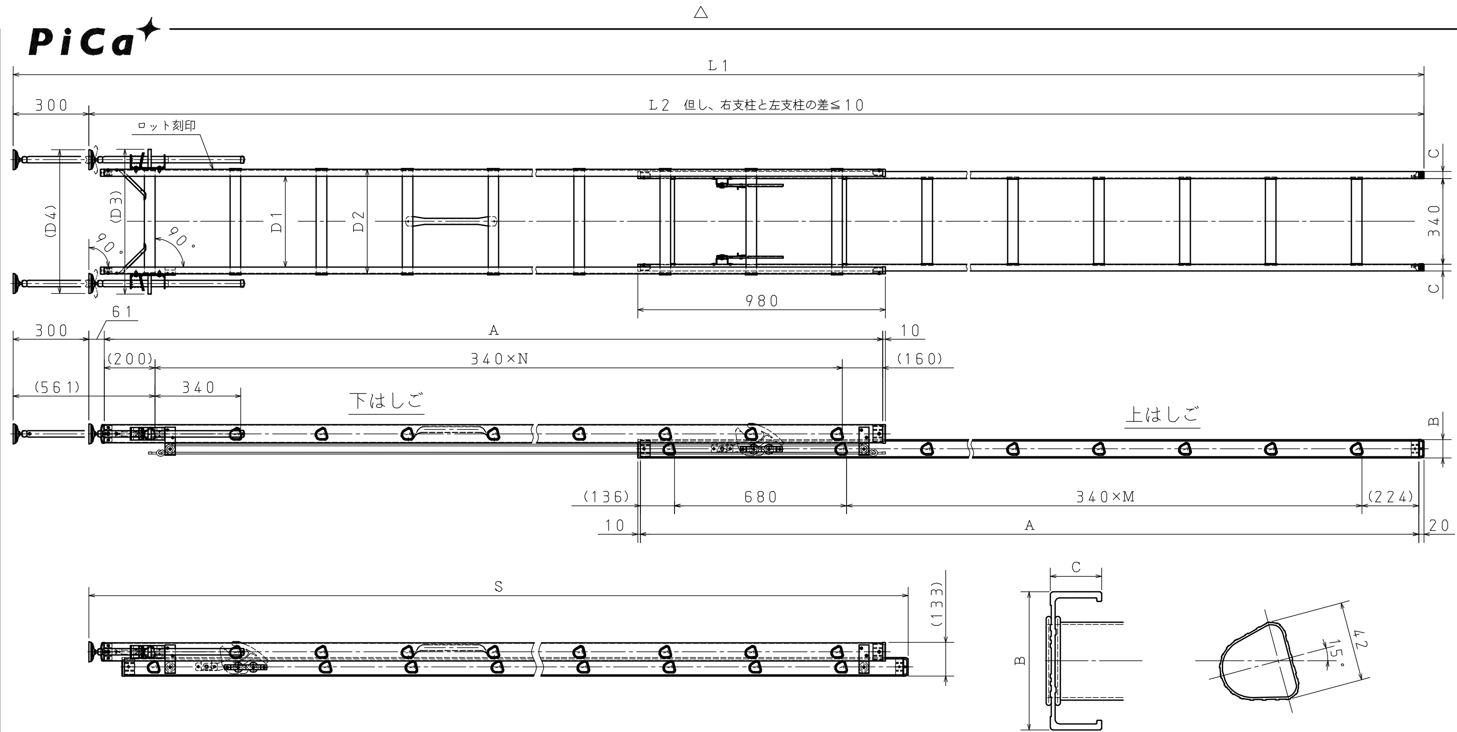
支柱及び踏ざん断面図 (S = 1 : 2)
