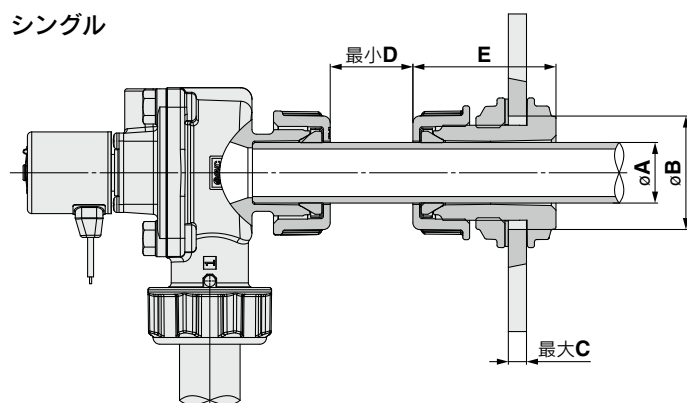
寸法表 (mm)
