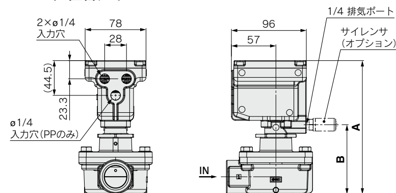
寸法表
