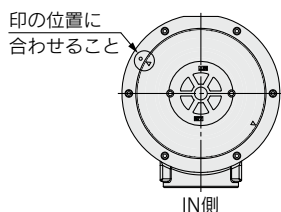
口径14サイズ 主弁配置
