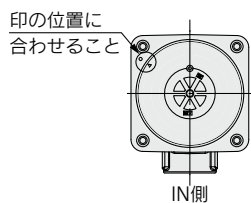
口径06・10サイズ 主弁配置
