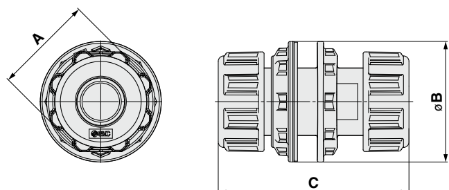
寸法表 (mm)
