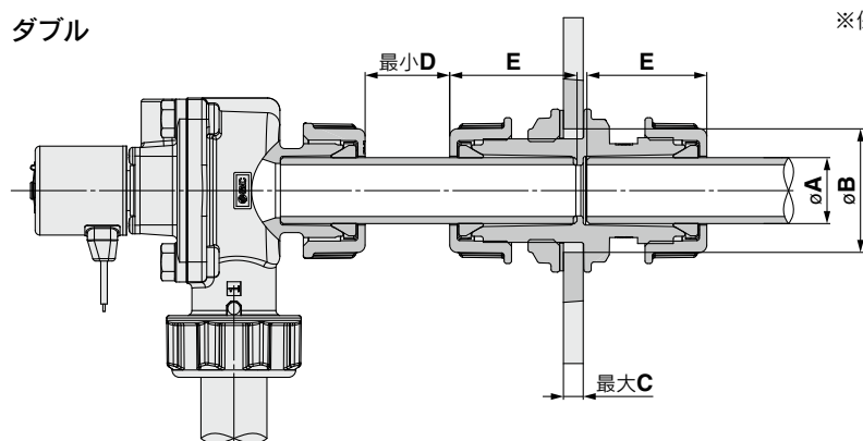
寸法表 (mm)
