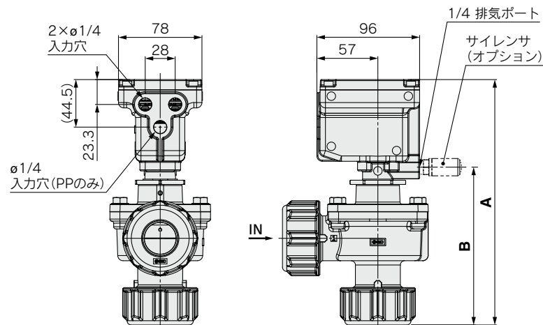
寸法表
