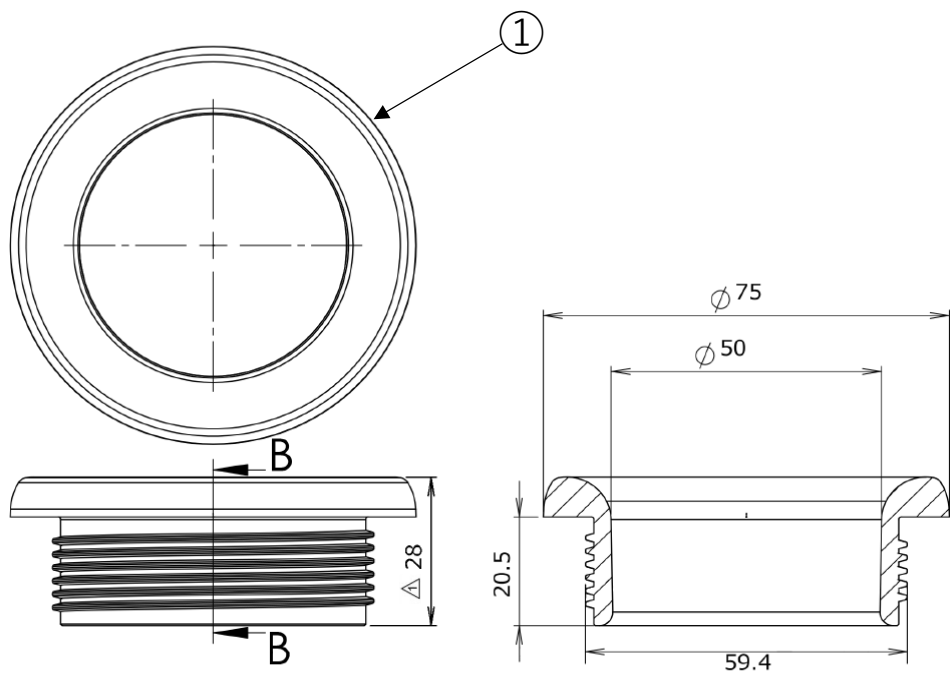
断面図 B-B
