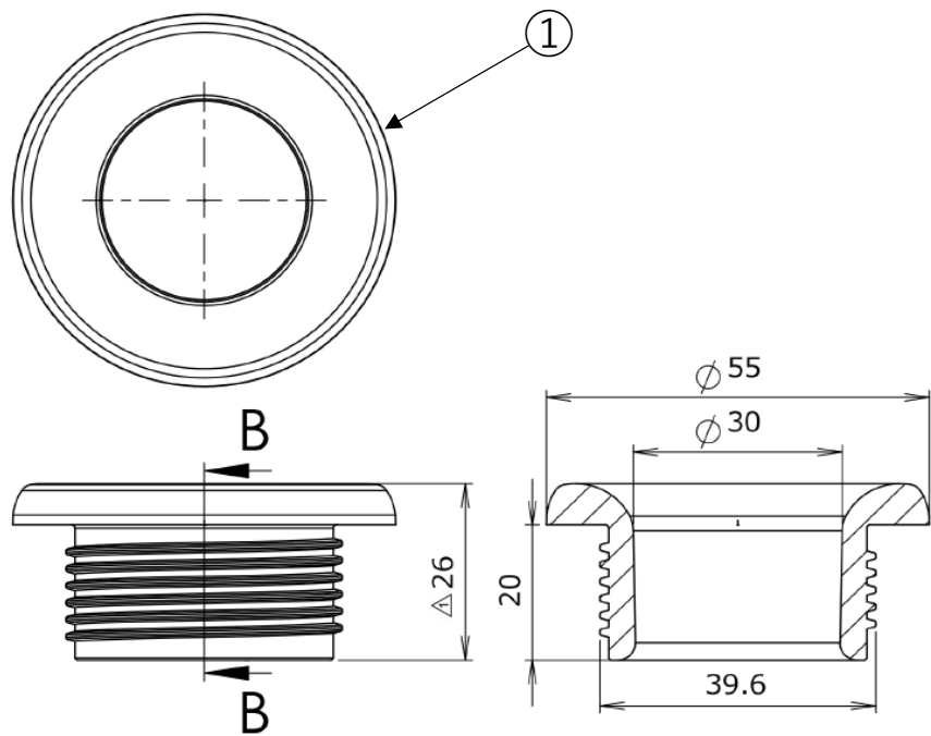
断面図 B-B
