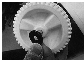
③④ワッシャを入れて、 ③⑤止めピンで止める。
