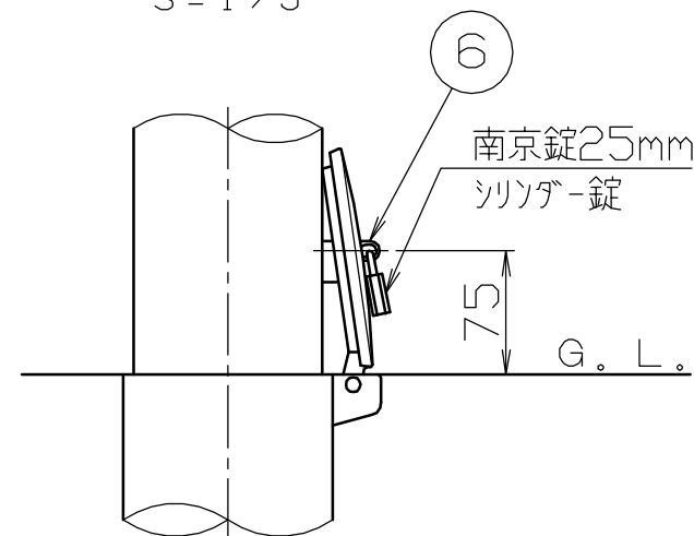
施錠部詳細図 S = 1 / 5
