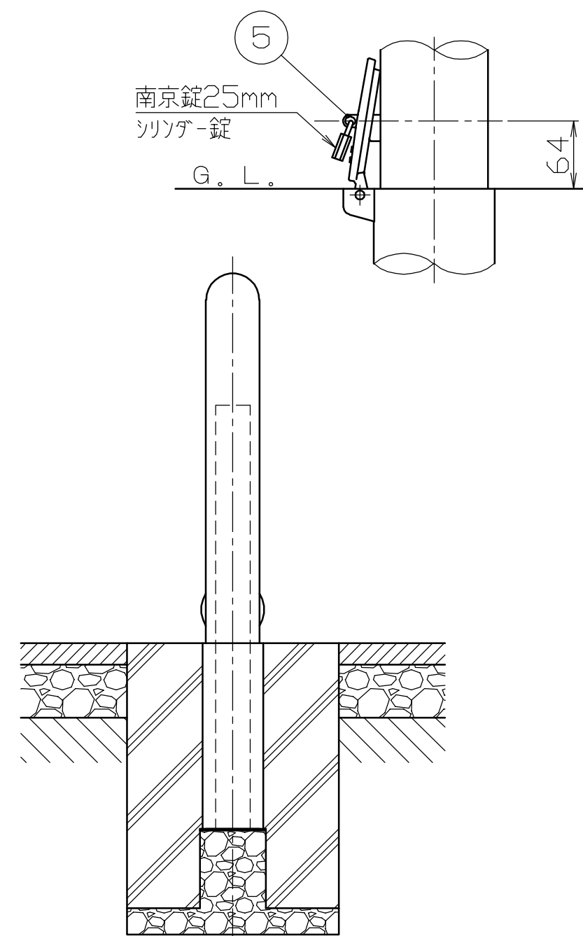
施錠部詳細図 S = 1 / 5
