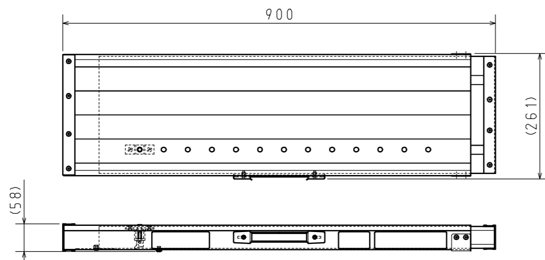
収納状態図
