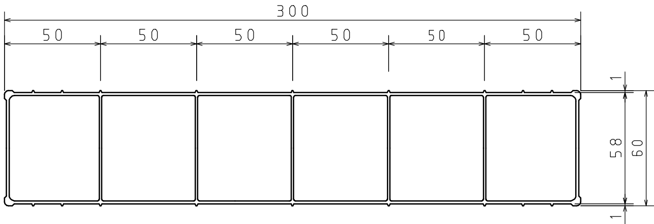
足場板断面図 (S = 1 : 2)
