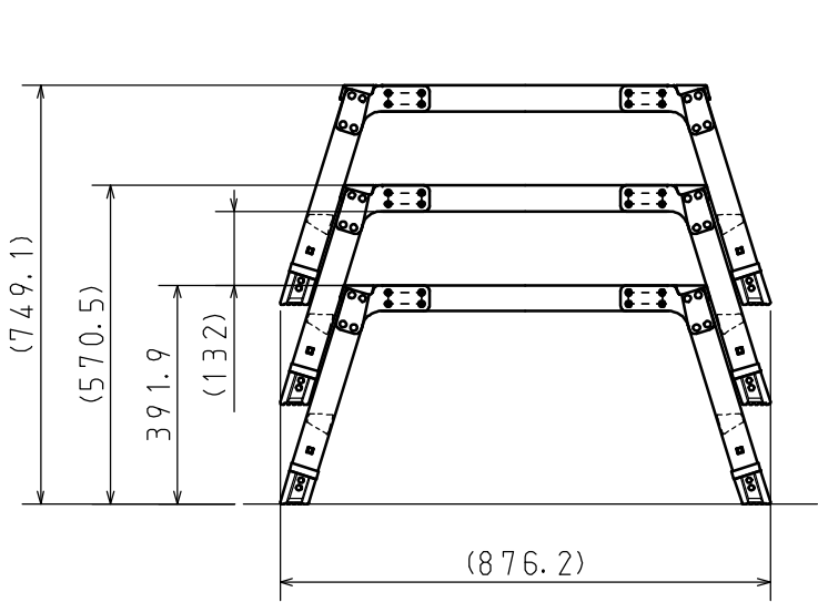
保管時積み重ね状態参考図（3台） S = 1 : 15
