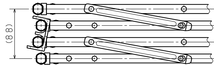
A-A断面 S = 1 : 4
