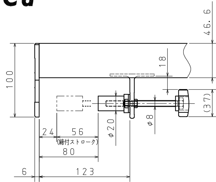
A部詳細図 (S = 1 : 3)
