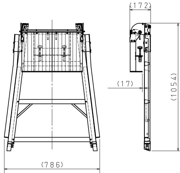
収納状態図
