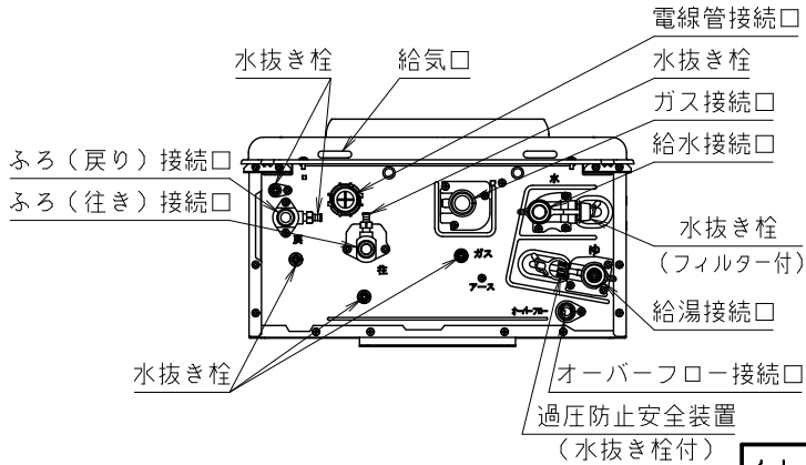
■底板よりの各接続口高さ(mm)
