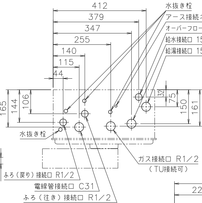
（機器上方よりの透視図）
