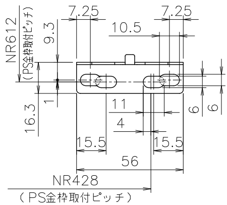
■D部詳細図（尺度1／2）
