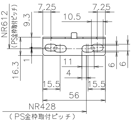
■D部詳細図（尺度1／2）
