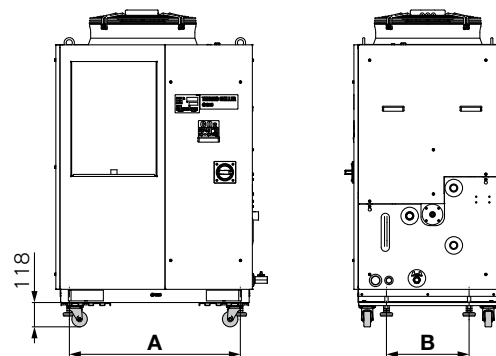
図1 取付状態
