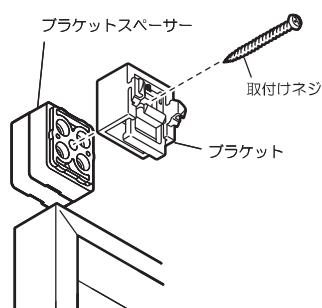
ブラケットスペーサー(22)の場合
