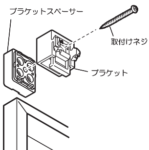
ブラケットスペーサー(12)の場合
