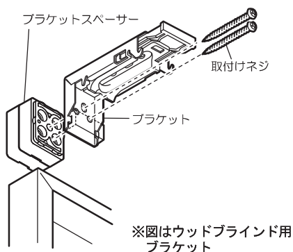
ブラケットスペーサー(22)の場合
