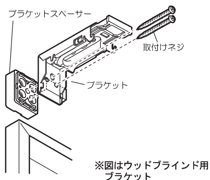
ブラケットスペーサー(12)の場合
