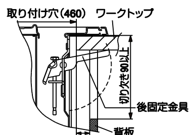
側面図
