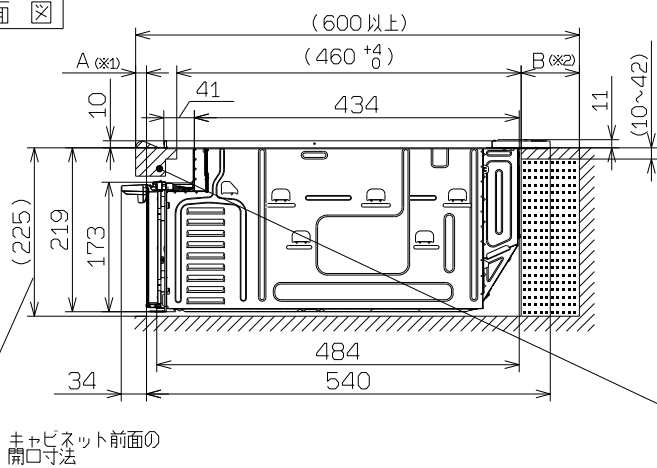
側面図
