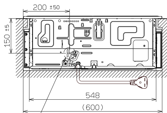
背面図
