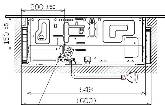
背面図
