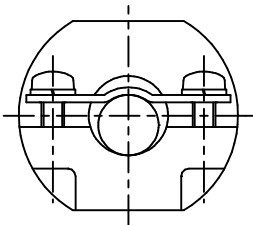
サイズ：16 パッキンNo.1~3 ケーブル径：φ6.0~12.0
