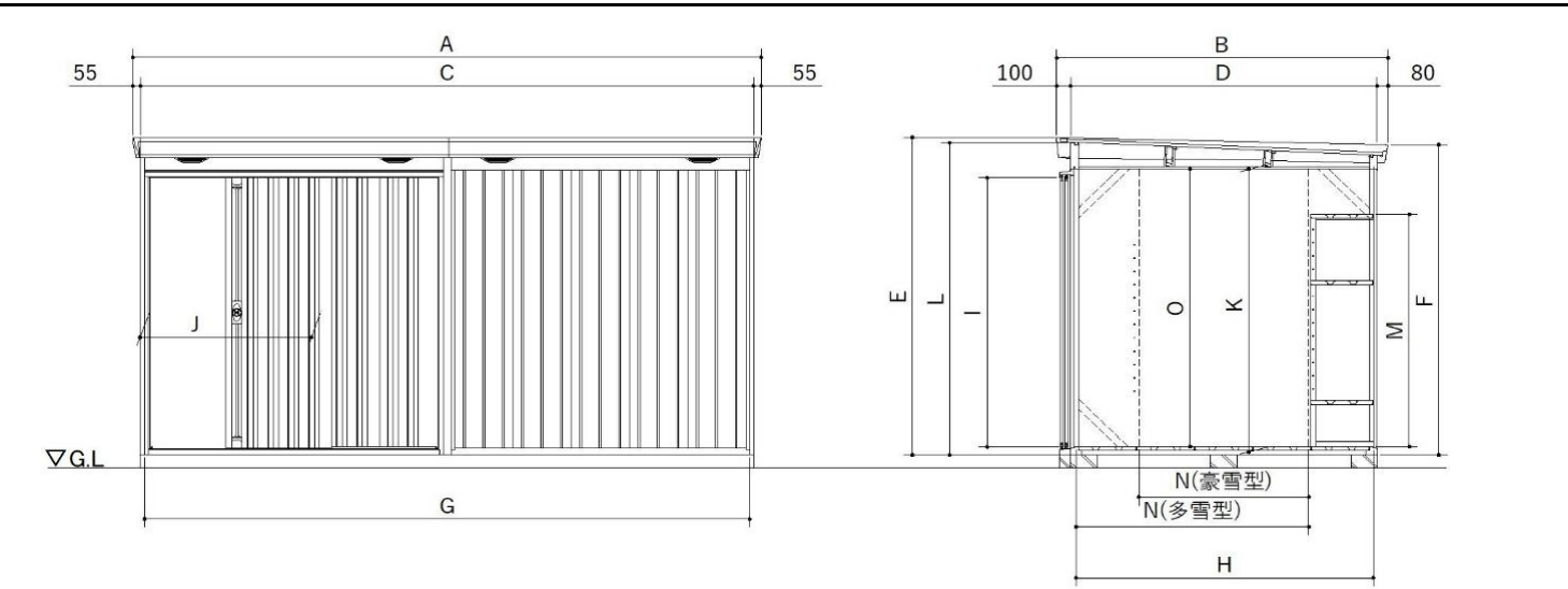
詳細寸法表(間口3580mm～5260mm)
