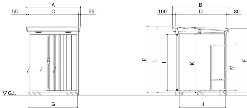
詳細寸法表(間口1370mm～1530mm)
