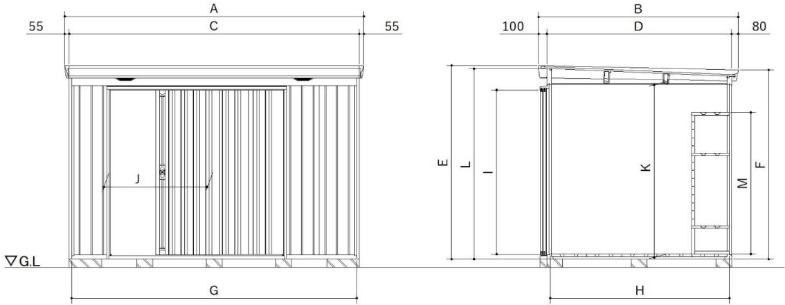
詳細寸法表(間口3540mm)
