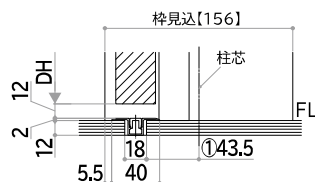
沓摺取付位置
