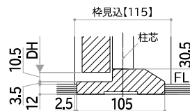
基本寸法表
