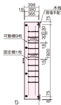
B-B断面図
