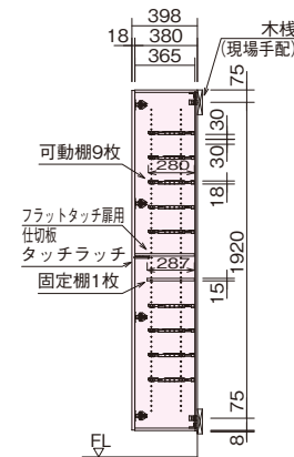
B-B断面図
