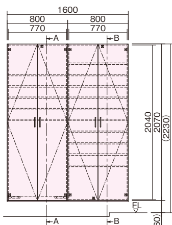
正面図
