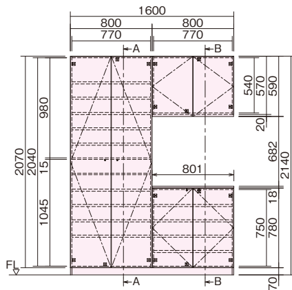
正面図
