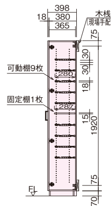
A-A断面図
