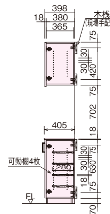
B-B断面図
