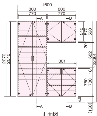
正面図
