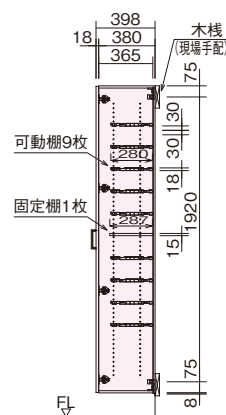
A-A断面図
