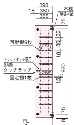
A-A断面図
