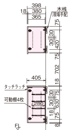
B-B断面図
