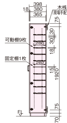
A-A断面図
