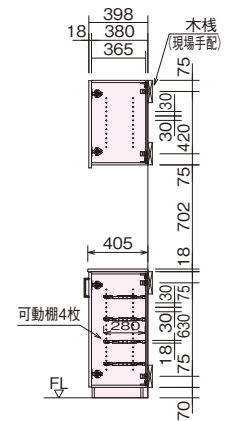
B-B断面図
