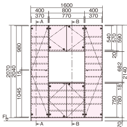
正面図
