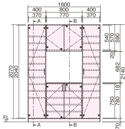
正面図
