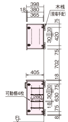
B-B断面図
