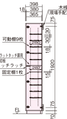
A-A断面図
