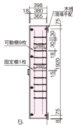
A-A断面図
