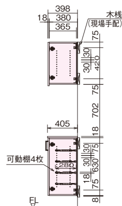
B-B断面図
