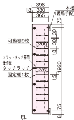
A-A断面図
