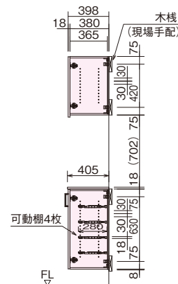
A-A断面図
