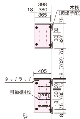
A-A断面図
