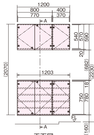
正面図
