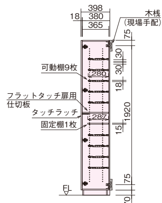
A-A断面図
