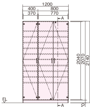
正面図
