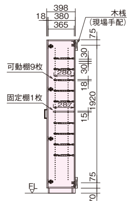
A-A断面図
