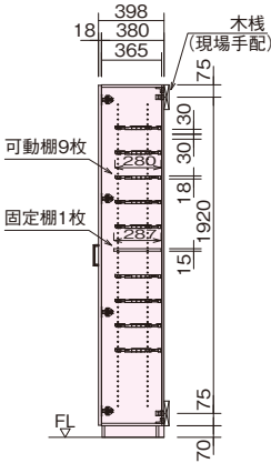
A-A断面図
