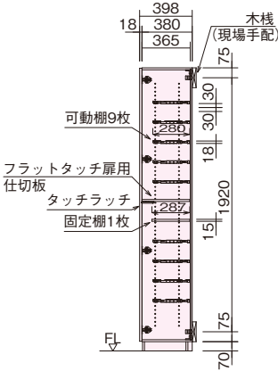
A-A断面図
