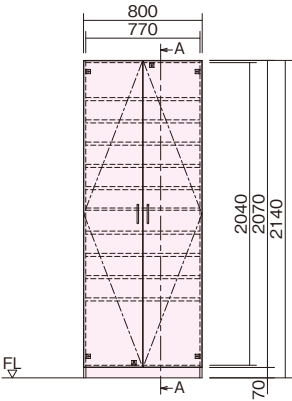
正面図
