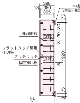
A-A断面図
