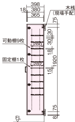
A-A断面図
