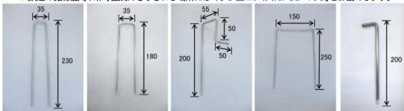
【角 U 型ピン】
