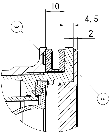
詳細 B S=1:1
