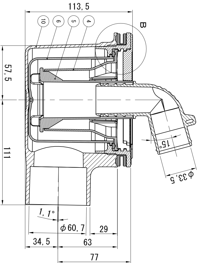
断面 A-A
