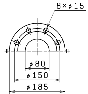
FLANGE SIZE フランジ寸法
