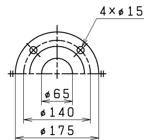
FLANGE SIZE フランジ寸法
