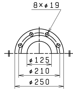
FLANGE SIZE フランジ寸法
