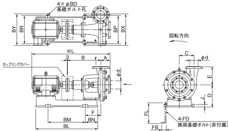
■据付外形寸法図（例） 単位：mm (口径40～100mm)
