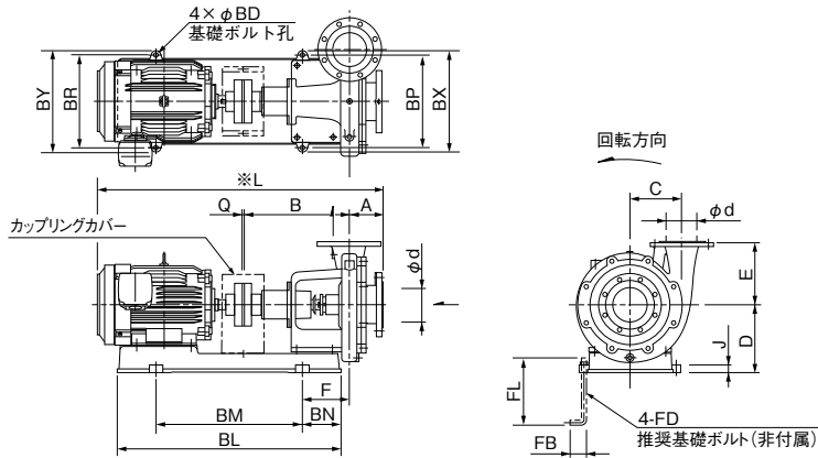
■据付外形寸法図（例） 単位：mm (口径125～150mm)
