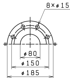
FLANGE SIZE フランジ寸法
