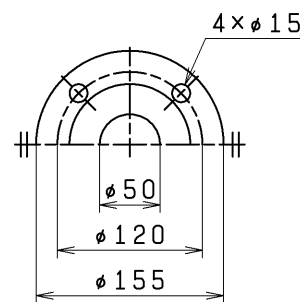
FLANGE SIZE フランジ寸法
