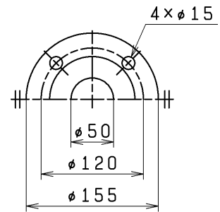
FLANGE SIZE フランジ寸法
