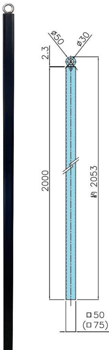
親綱支柱 (M12用 SUSアイボルト付き)
