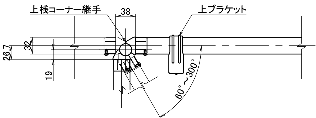
コーナー 継手部納り図 S:1/4
