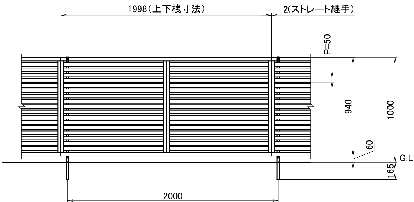
ストレート継手部納り図 S:1/4
