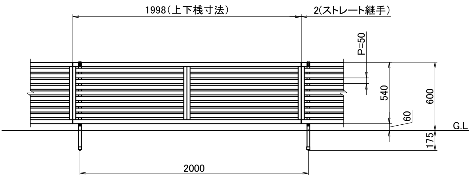
ストレート継手部納り図 S:1/4
